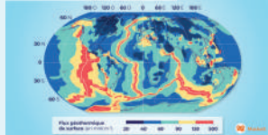
Carte mondiale du flux géothermique surfacique
